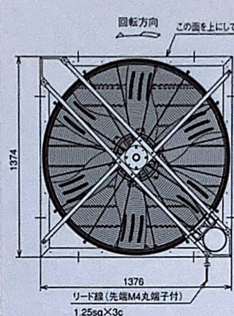
FGX1370NA
